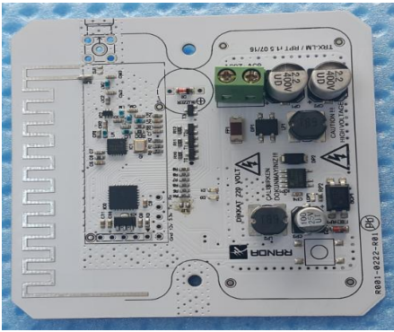
Şekil 5 : PCB Kartı ön yüzü.
