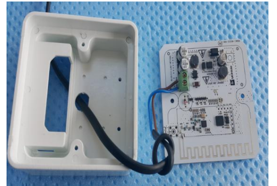
Şekil 7 : Güç bağlantısı yapılır.
