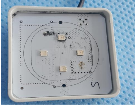
Şekil 8 : PCB kartı alt kapağa yerleştirilir.
